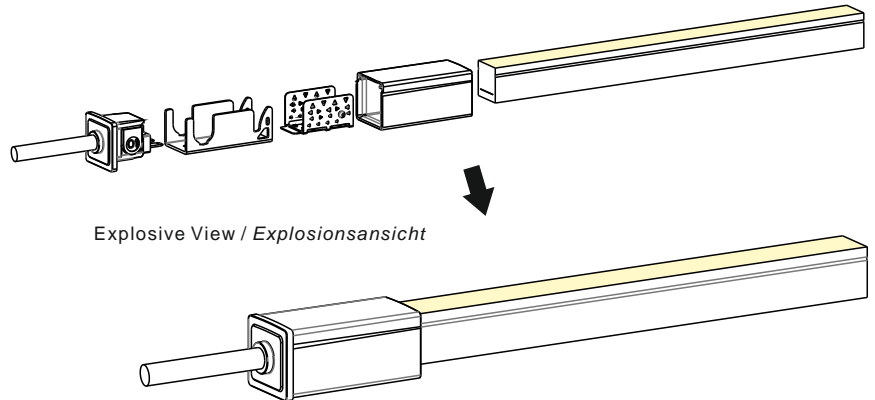
Finished Assembly View / Ansicht zusammengebaut.
